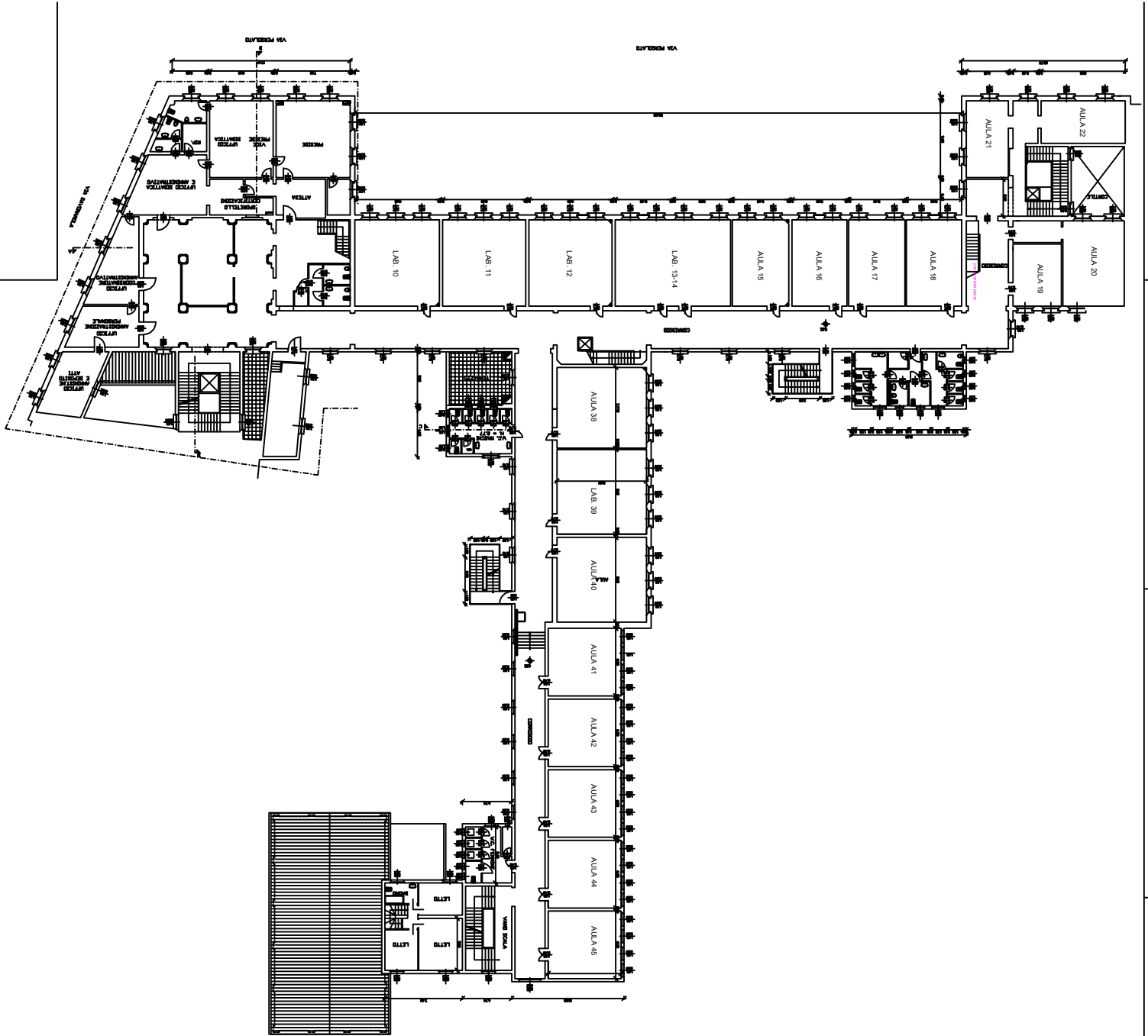
PIANTA PRIMO PIANO VARIANTE SCALA 1:100
