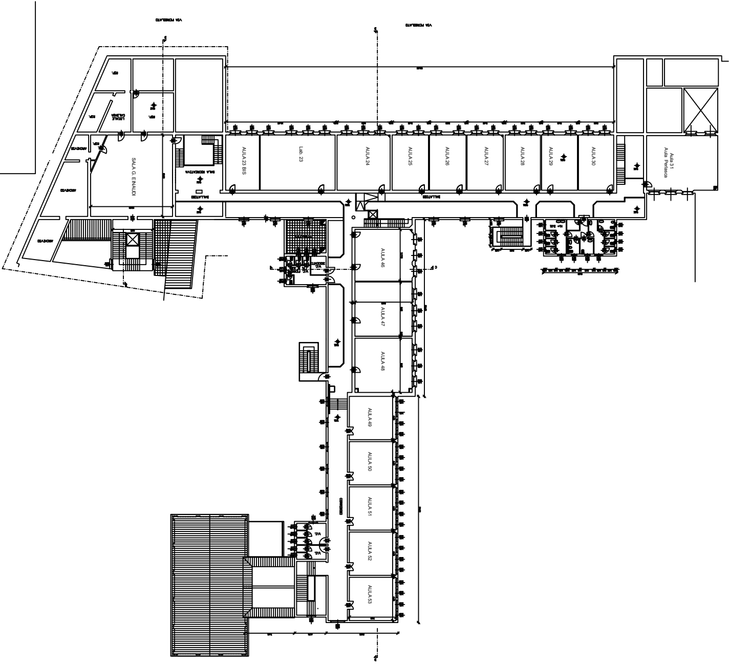
PiANTA SECONDO PIANO VARIATO SCALA 1:100
